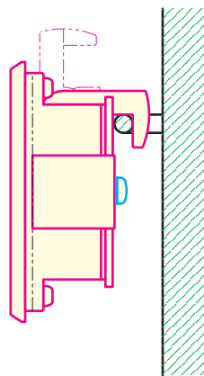
取り付け時断面
